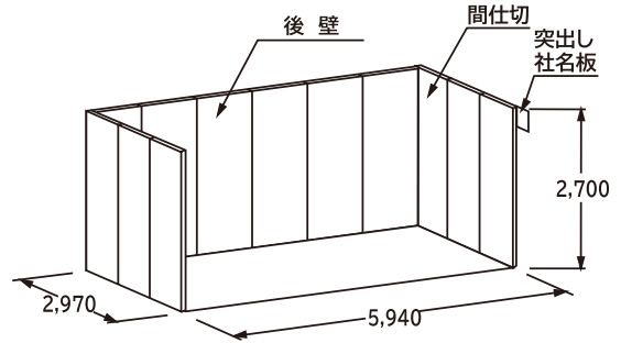
【例:2小間の場合】 (W5,940×D2,970×H2,700mm)
